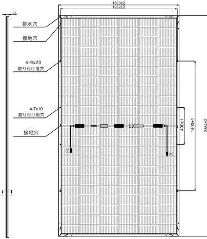
太陽光発電モジュール図面 単位: mm
